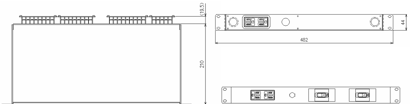
【NFB-T5 外観図】
