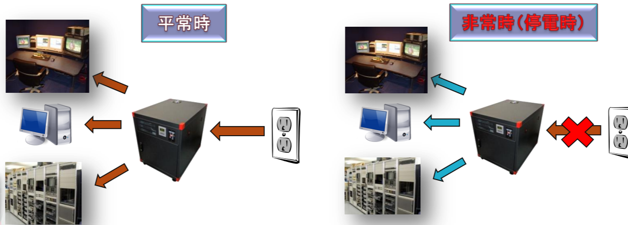
LIB-6400はUPS機能により停電など非電源供給時には6400Whの大容量バッテリーから電気供給し長時間の運用が可能です。(500Wで約10h運用可能)
