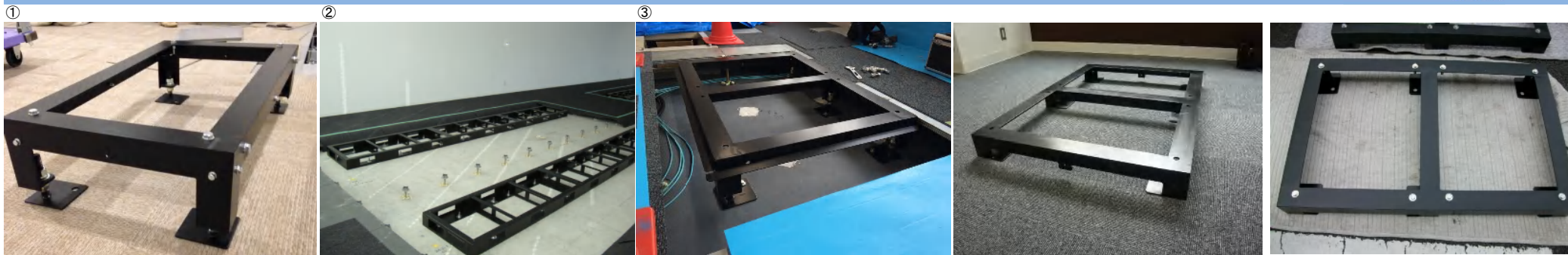
【ジャッキアップ式 ラック単体仕様】 参考サイズ:W=700mm/H=500mm/D=1000mm 標準価格:100,000- (税抜き) *フリーアクセスパネル受けアングル無し 【ダイス型(板材板金)式 ラック3連仕様】 参考サイズ:W=1640mm/H=80mm/D=650mm 標準価格:190,000- (税抜き) *写真は上記架台を1列あたり3連結しております。 【ジャッキアップ式 ラック2連仕様】 参考サイズ:W=1140mm/H=200mm/D=710mm 標準価格:180,000- (税抜き) *フリーアクセスパネル受けアングル(上下調整機構付き:4本/1式)標準装備 【コタツ式 ラック2連仕様】 参考サイズ:W=1140mm/H=100mm/D=810mm 標準価格:150,000- (税抜き) ライナー敷設タイプ/フリーアクセス受けアングル無 【ジャッキアップ式 ラック2連仕様】 参考サイズ:W=1140mm/H=150mm/D=710mm 標準価格:170,000- (税抜き) ジャッキアップ式/フリーアクセス受けアングル無
